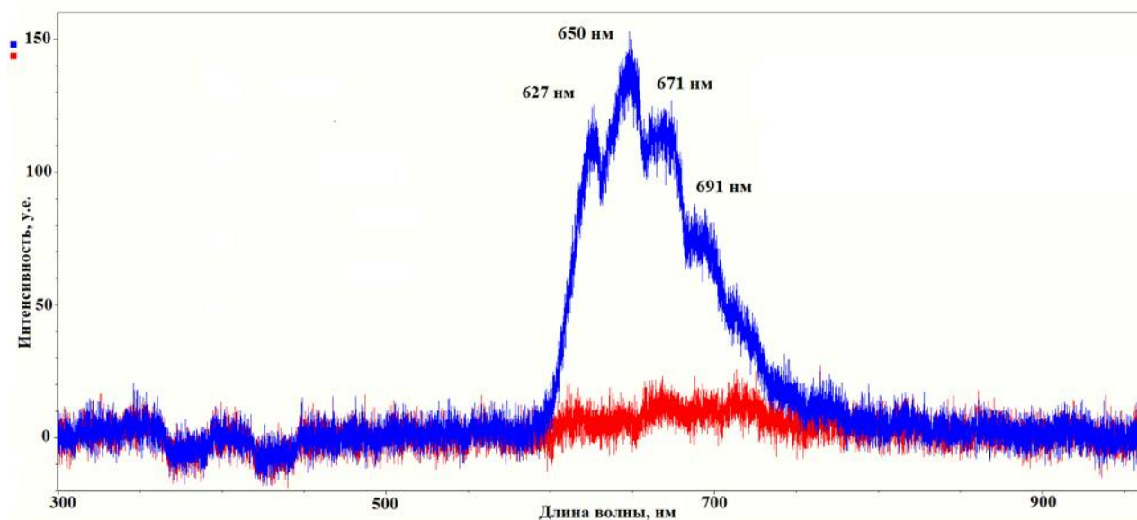
Рис. 1. Спектр излучения от «белого» светодиода, прошедшего через палец человека: синий график — палец не перетянут эластичным жгутом; красный график — палец перетянут эластичным жгутом, и свет через него не проходит
